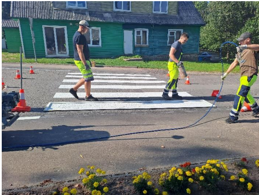
1 pav. Pėsčiųjų perėjos įrengimas
